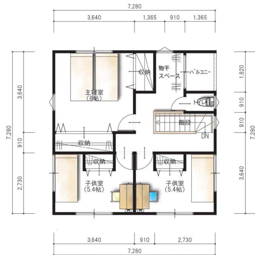
2階平面図
